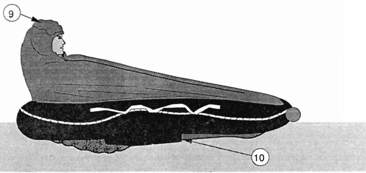
Figur 5. Teckning av Mk 10 med flotte. 1. CO 2 -flaska för fyllning av flytring. 2. Länstrut. 3. Slang för luftpåfyllnad av uppblåsbar botten. 4. Slang för luftpåfyllnad av flytring. 5. Uppblåsbar del av flottens botten. 6. Undanfälld utstigningshuva. 7. Ficka för hopvikt flotte. 8. HIS (hood-inflation system)-slang. 9. Stänkskydd (uppfällt). 10. Fast drivankare.
